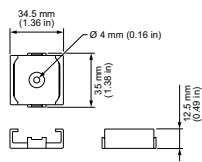
Spacer
