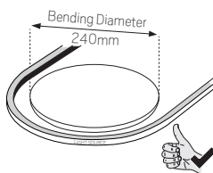
LEDSTRIP 24V NEON TOP IP67
