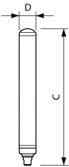
Tforce SOX G2 4000lm B22 840 50K
