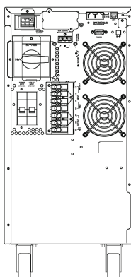
MSIII 6000
