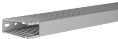
SLISSET LEDNINGSKANAL,85x31mm
