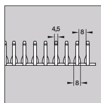
Sidestansing VK flex 20, 30 og 40
