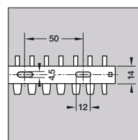
Bunnstansing VK flex 20 og 30
