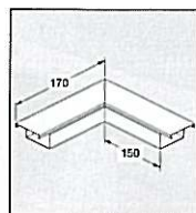
Flatvinkel Bestillingsbetegnelse
