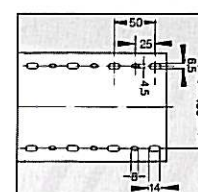
Bunnstansing
