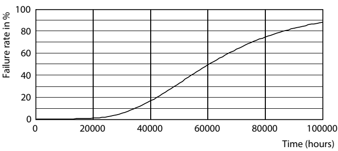
LEDtube_60K
