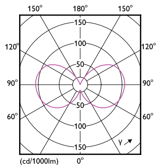
LEDluster MAS P45 3,4W E14 927 CL-LDD
