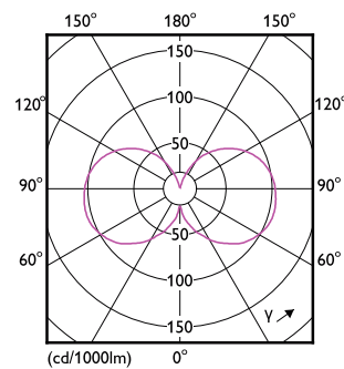
LEDcandle MAS SLR B35 3,4W E14 927 CL-LDD
