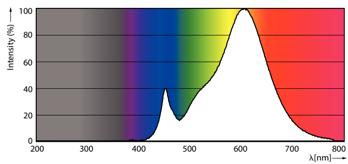
LEDlustrer CorePro 2,8W P45 E27 827 FR-POC
