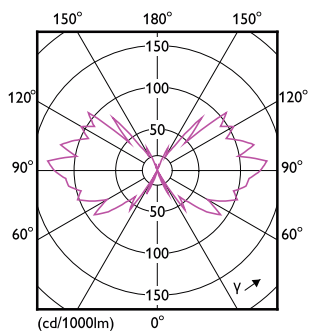
LEDbulb SLR Crystal 7W E27 818 Smoky-LDD
