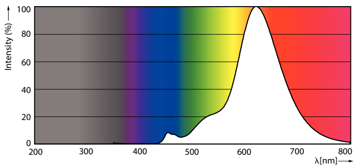
LEDbulb SLR 7W Crystal E27 818 Smoky-POC
