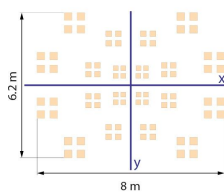
Deteksjonsmønster på gulvnivå ved 2,5 m monteringshøyde
