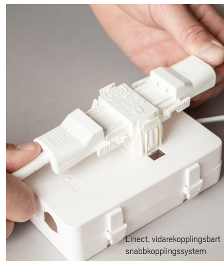
Linect, 3- och 5-polig för Wieland, Ensto, Wago/Winsta
