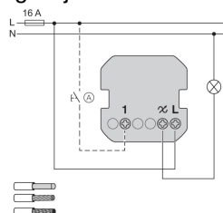
Koblingsskjema
