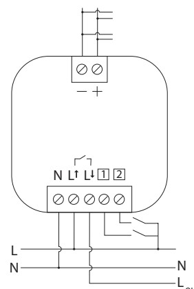
Kobling for 1-10 V buss (med avbrudd av forsyning til last)
