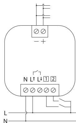
Kobling for 0-10 V buss (uten avbrudd av forsyning til last)
