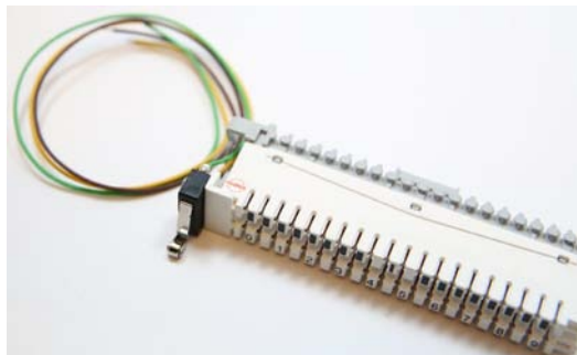
Bildet viser microbryter påmontert Molex DCN-plint
