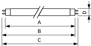
TL-D 18W/840
