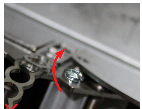
✗ Falsch / Wrong / Faux Lasche behindert die Schraube. Schraube kann nicht wegtäuchen. / Metal strap not bent back inhibits the screw movement. / La patte n'est pas repliée et gêne le mouvement de la vis.
