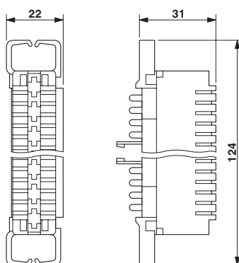
Målskisse
