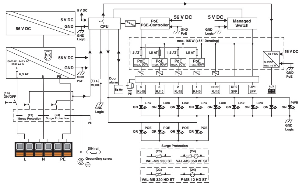
Koblingskjesma
