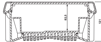
Målskisse
