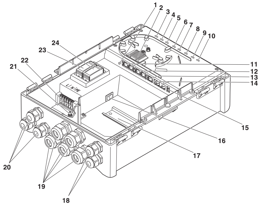
Skjemategning
