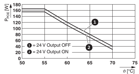
Derating (samlet PoE-ytelse)
