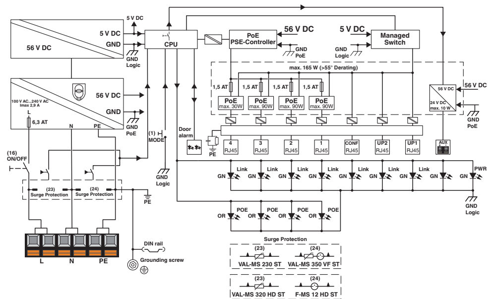
Koblingsskjema
