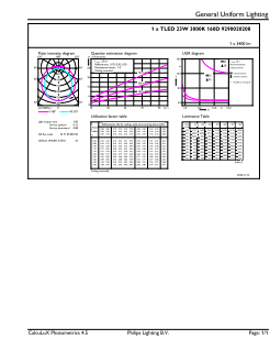
TLED_5ft_220-240V_23-58W_3400lm_3000K_G13
