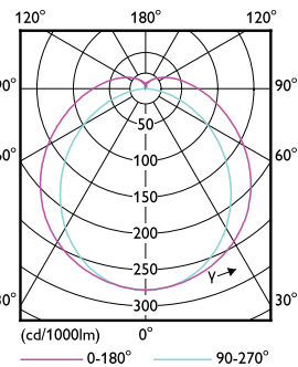
TLED_5ft_220-240V_23-58W_G13
