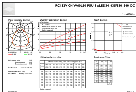
IFGU1_RC132VG4W60L60PSU1xLED34_43S830_840OC
