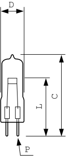
7158XHP 150W G6.35 24V
