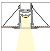
Montage med fjäderfäste
