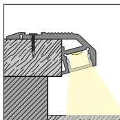
Montage på steg med skruvar
