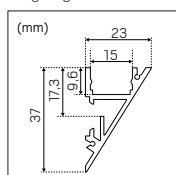
Uppljus med dolt fäste och ledningsdragning
