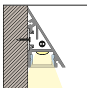
Nerljus med dolt fäste och ledningsdragning
