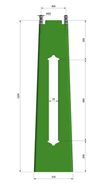
Ørstafundament c/c 200mm, H=1250 mm
