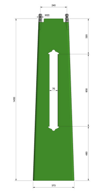
Ørstafundament c/c 240mm, H=1500 mm
