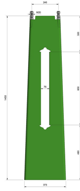
Ørstafundament c/c 240mm, H=1500 mm
