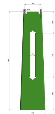
Ørstafundament c/c 240mm, H=1500 mm
