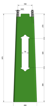
Ørstafundament c/c 160mm, H=1000 mm
