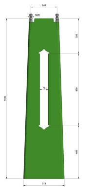
Ørstafundament c/c 240mm, H=1500 mm
