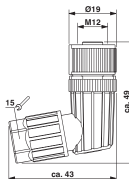
Målskisse
