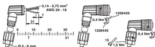
Funksjonstegning
