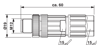
Målskisse
