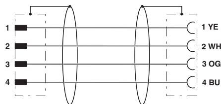
Koblingsskjema
