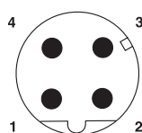
Polskisse plugg M12, 4-polet, D-kodet, stiftside
