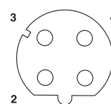
Polskisse bøssing M12, 4-polet, D-kodet, bøssingside
