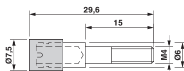
Målskisse
