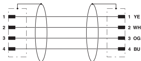
Koblingsskjema
