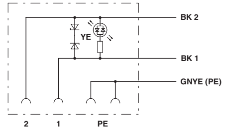
Ventilpluggens kontakttilordning
