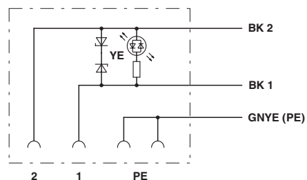
Ventilpluggens kontakttilordning
