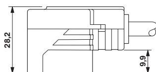
Ventilplugg, byggform A, sett fra siden
