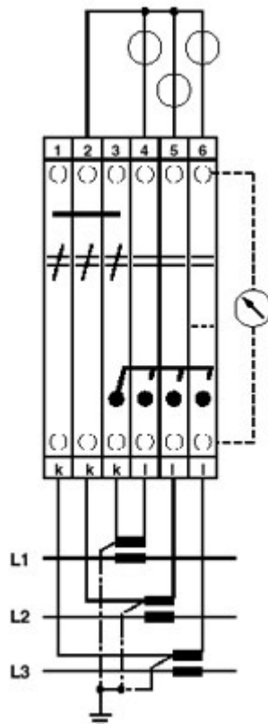
Skjemategning
