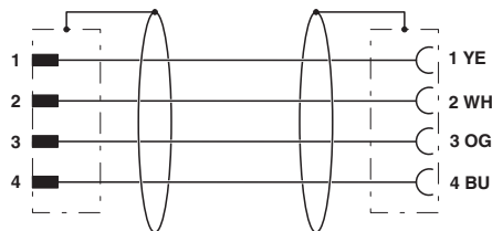
Koblingsskjema
