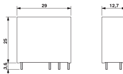
Målskisse
