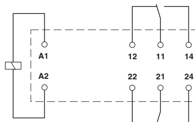
Koblingsskjema
