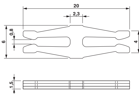
Målskisse
