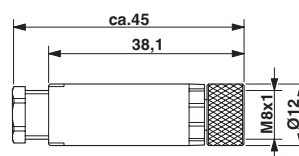
Målskisse
