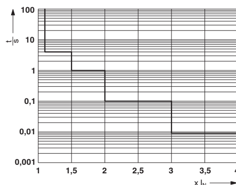
Utløsekarakteristikk
