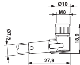
Målskisse
